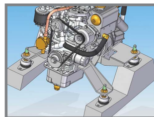
◦ SPESIALTILPASSEDE MOTORFESTER ◦
