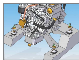
◦ SPESIALTILPASSEDE MOTORFESTER ◦
